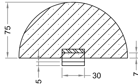
A-A'
